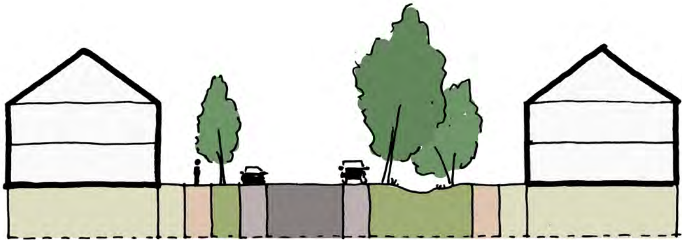
Profiel G : tweerichtingsweg hoofdonthut
